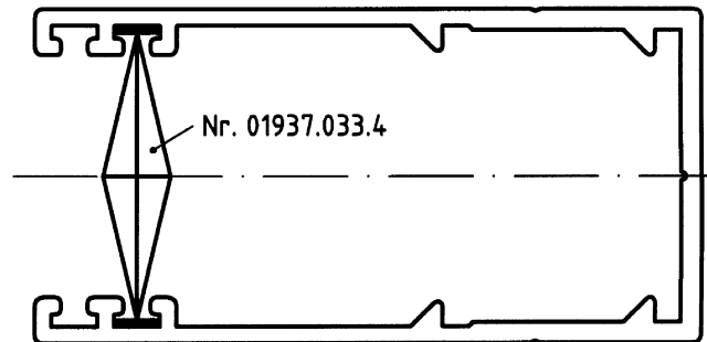
Führungsschiene 80×40mm, Nr. 02538.033.3
