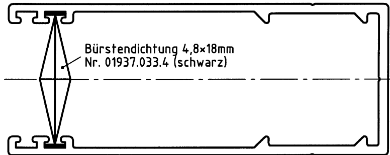
Führungsschiene 100×40mm, Nr. 12780.033.3
