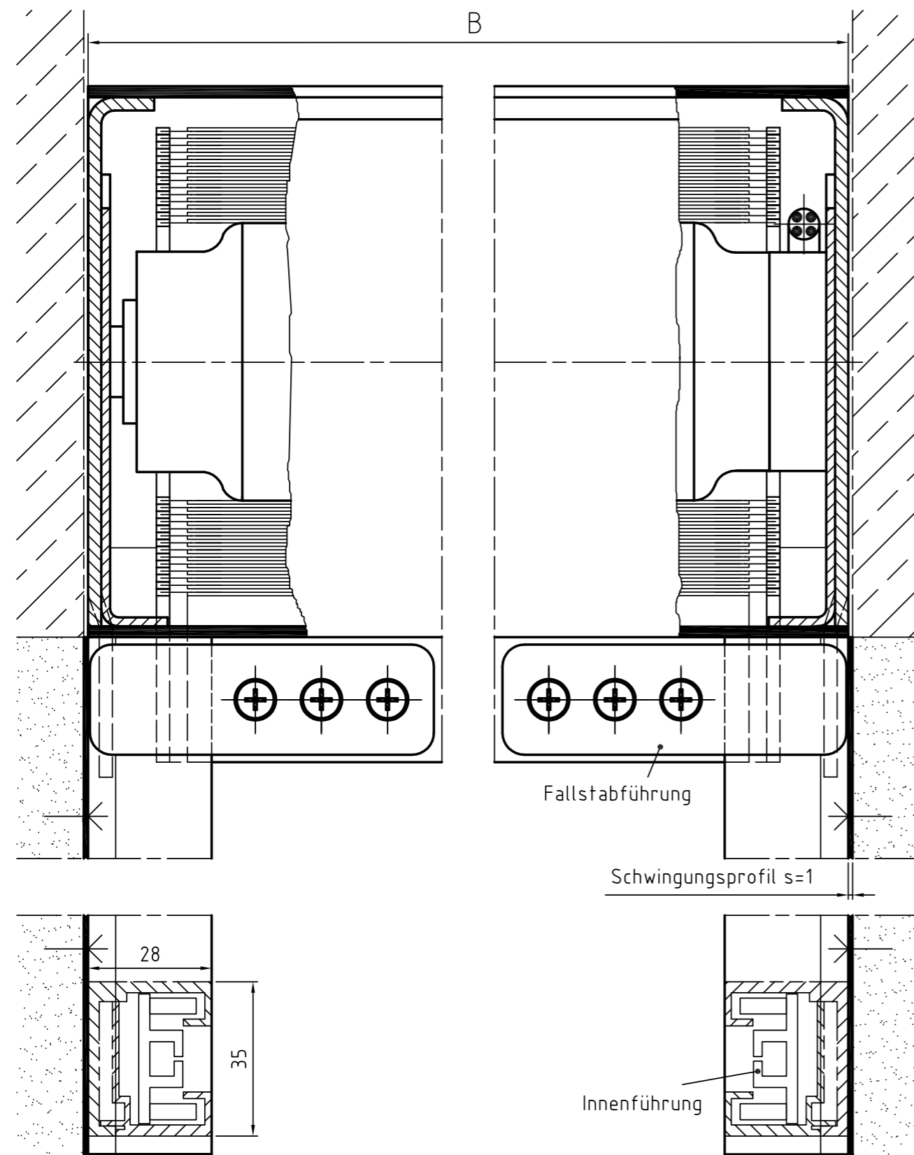
Zeichnung BS-ZIP-MQ1 – Querschnitt Systemskizze | ohne Maßstab | sämtliche Angaben in mm
