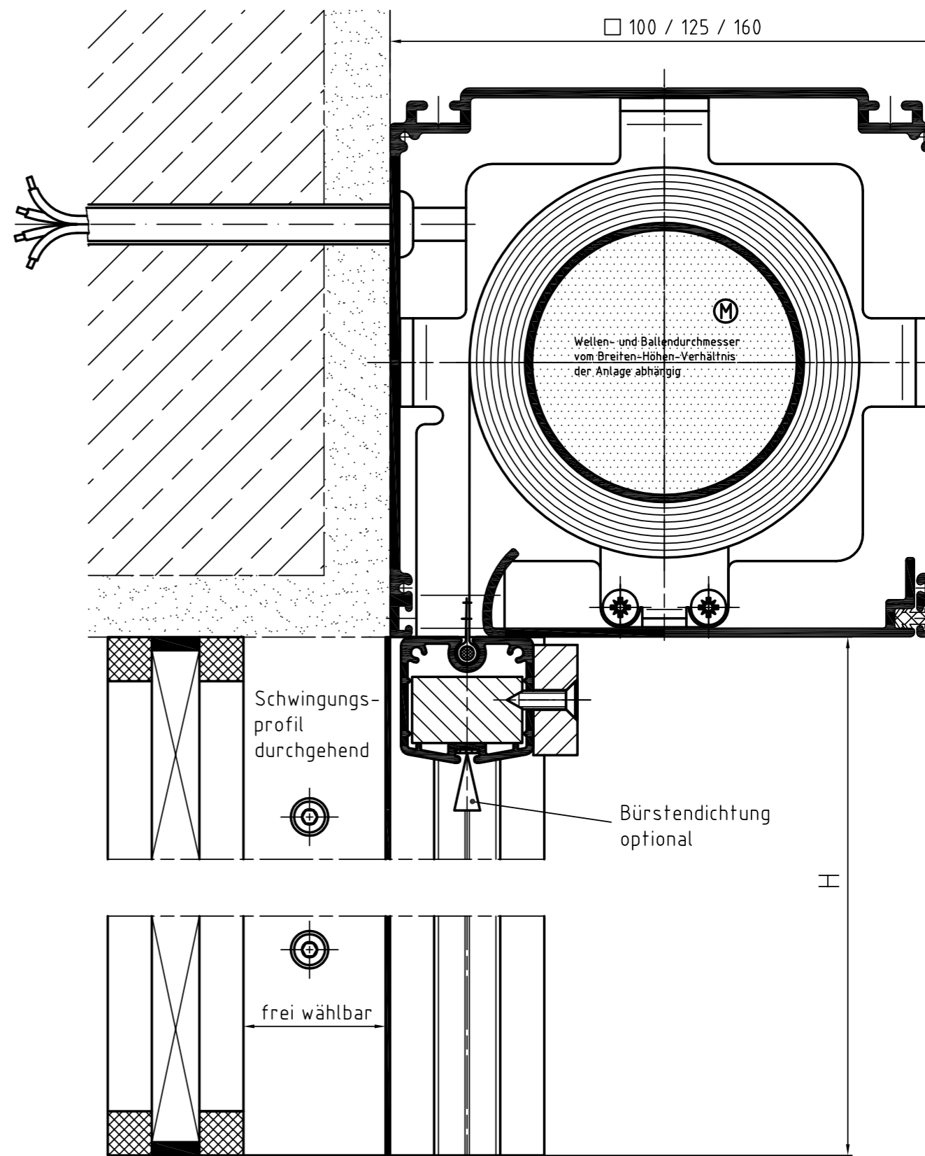
Zeichnung BS-ZIP-MQ1 – Längsschnitt Systemskizze | ohne Maßstab | sämtliche Angaben in mm
