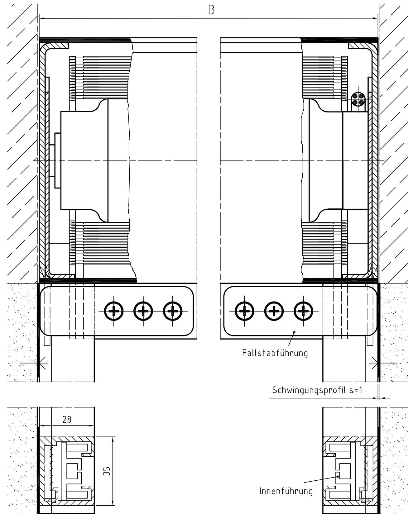
Zeichnung BS-ZIP-MQ2 – Querschnitt Systemskizze | ohne Maßstab | sämtliche Angaben in mm
