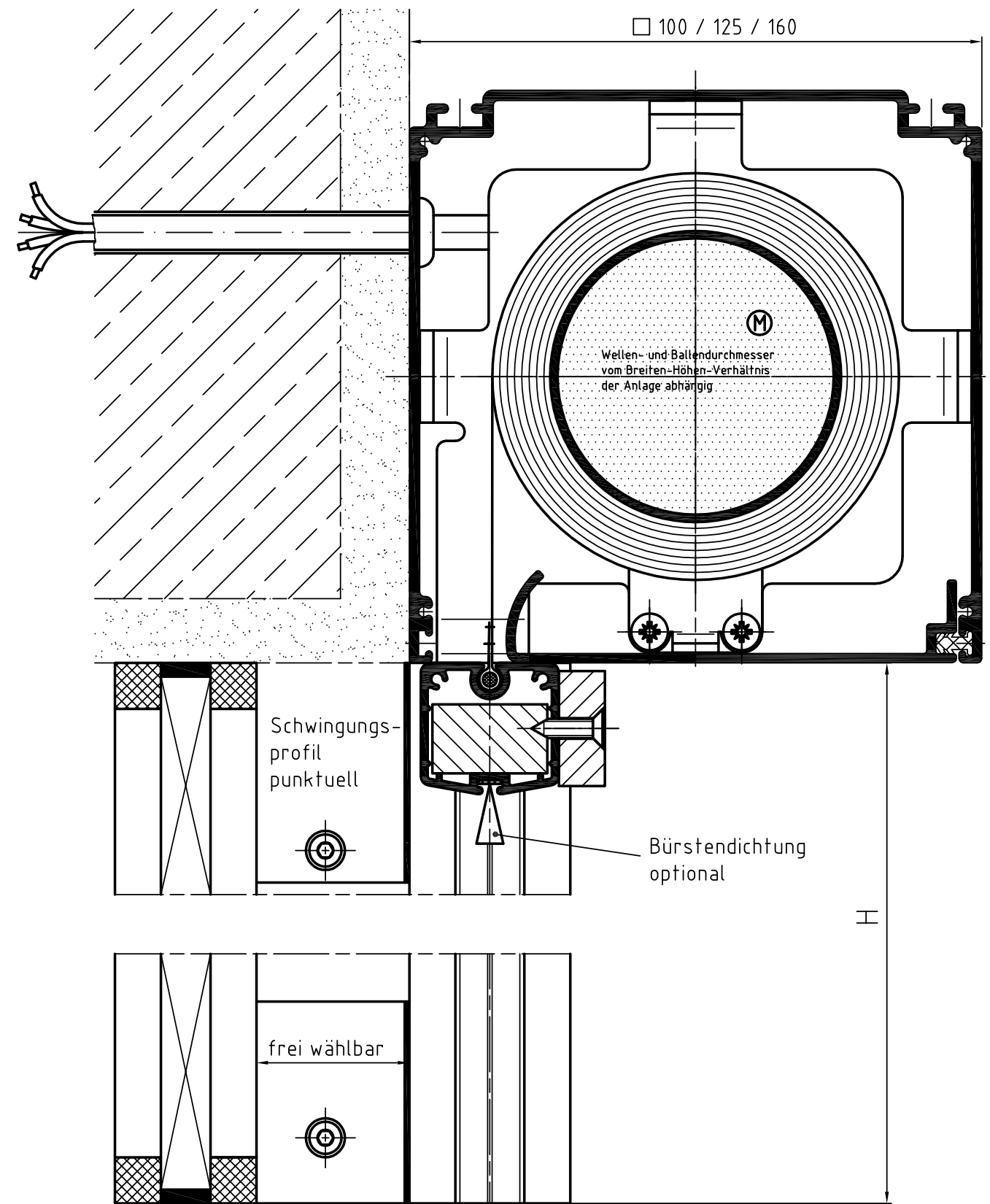
Zeichnung BS-ZIP-MQ2 – Längsschnitt Systemskizze | ohne Maßstab | sämtliche Angaben in mm
