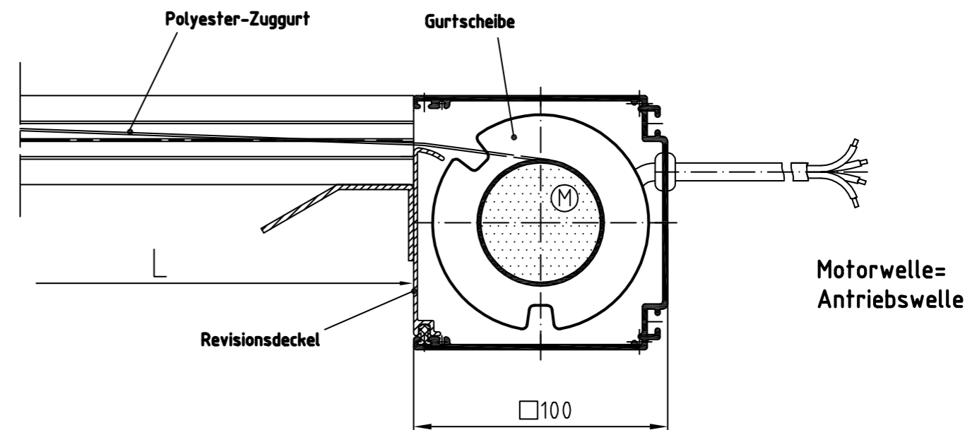
Zeichnung GZ-ZIP-MQ 100 – Längsschnitt Systemskizze | ohne Maßstab | sämtliche Angaben in mm
