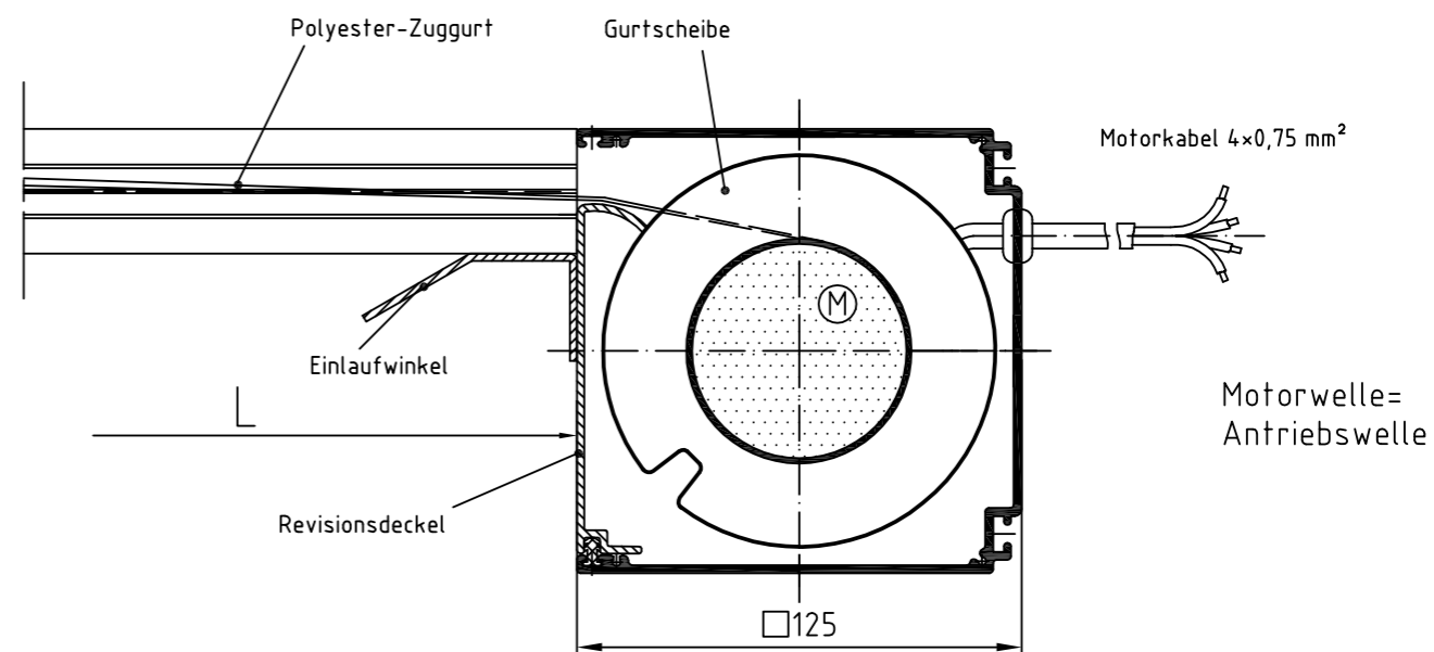
Zeichnung GZ-ZIP-MQ 125 – Längsschnitt Systemskizze | ohne Maßstab | sämtliche Angaben in mm
