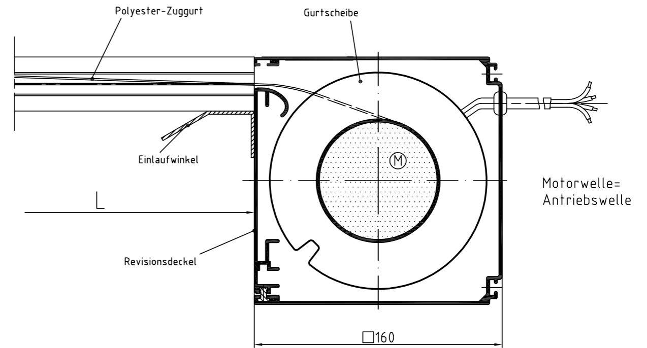
Zeichnung GZ-ZIP-MQ 160 – Längsschnitt Systemskizze | ohne Maßstab | sämtliche Angaben in mm
