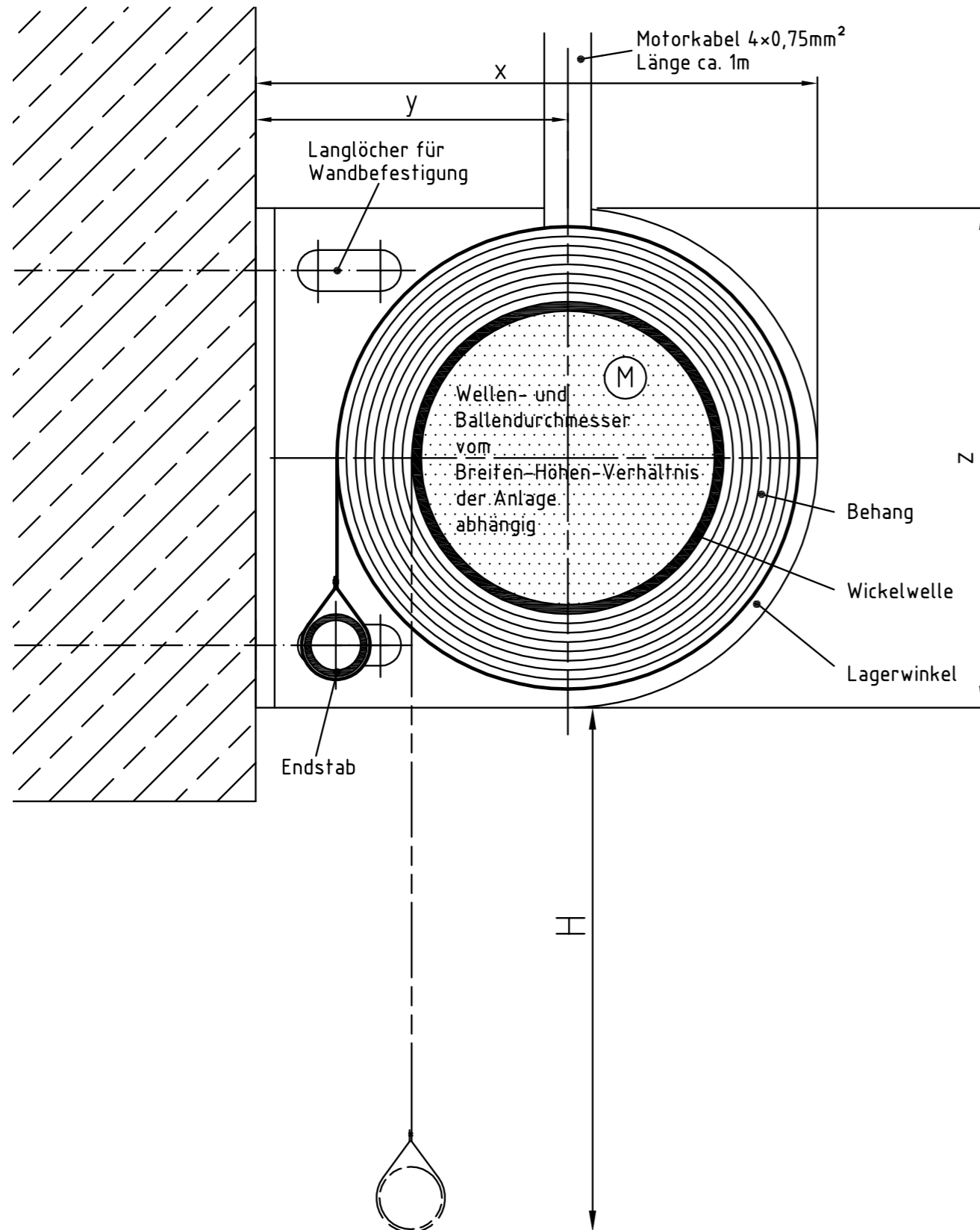
Zeichnung MO - Querschnitt Systemskizze | ohne Maßstab | sämtliche Angaben in mm
