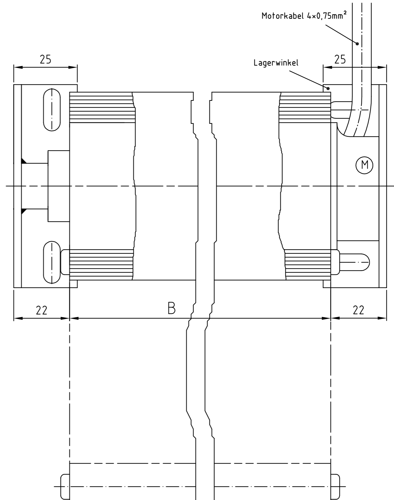
Zeichnung MO - Längsschnitt Systemskizze | ohne Maßstab | sämtliche Angaben in mm
