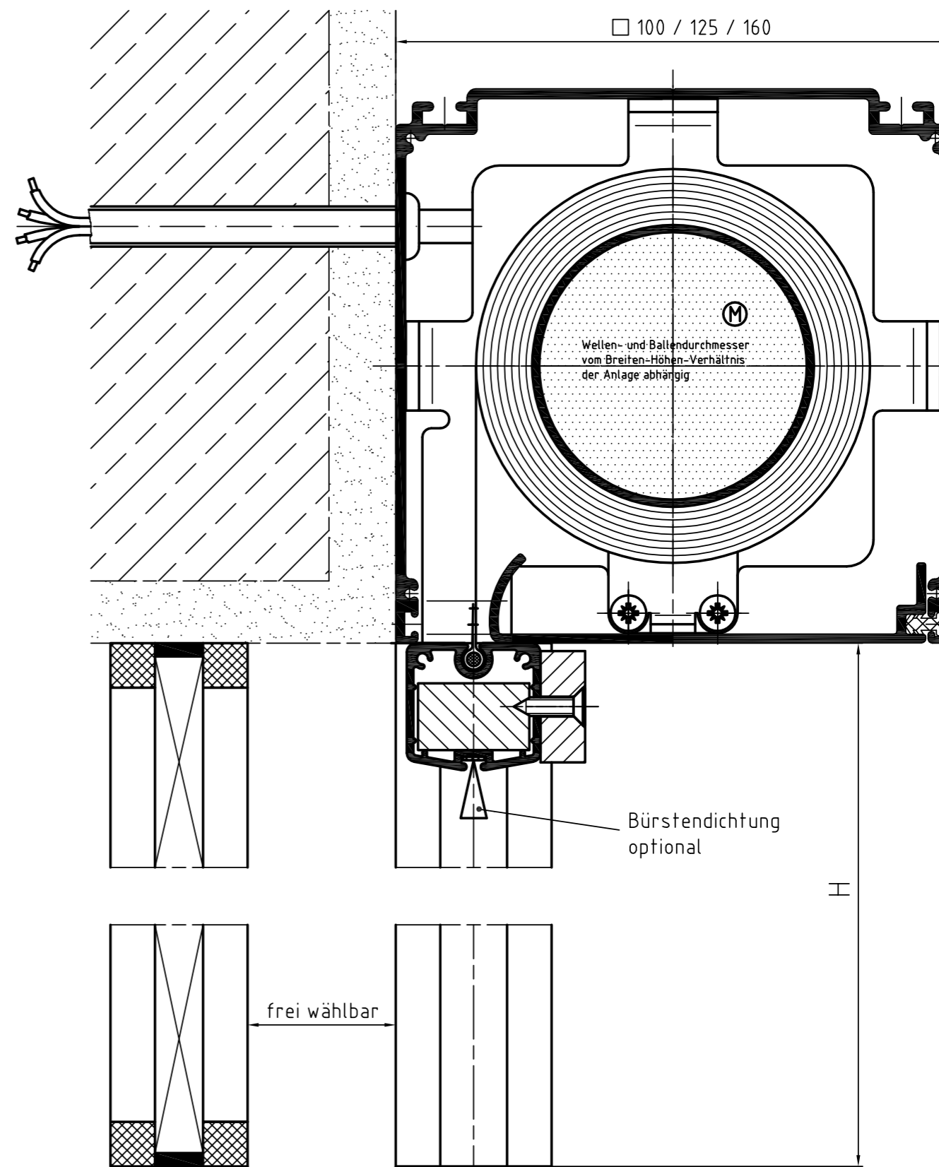
Zeichnung BS-C-MQ1 – Längsschnitt Systemskizze | ohne Maßstab | sämtliche Angaben in mm
