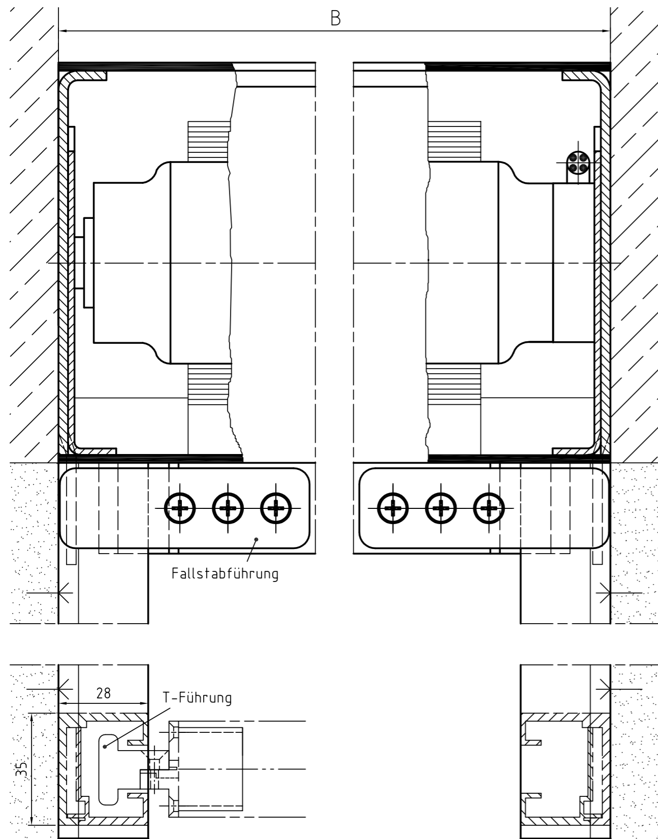
Zeichnung BS-C-MQ1 – Querschnitt Systemskizze | ohne Maßstab | sämtliche Angaben in mm
