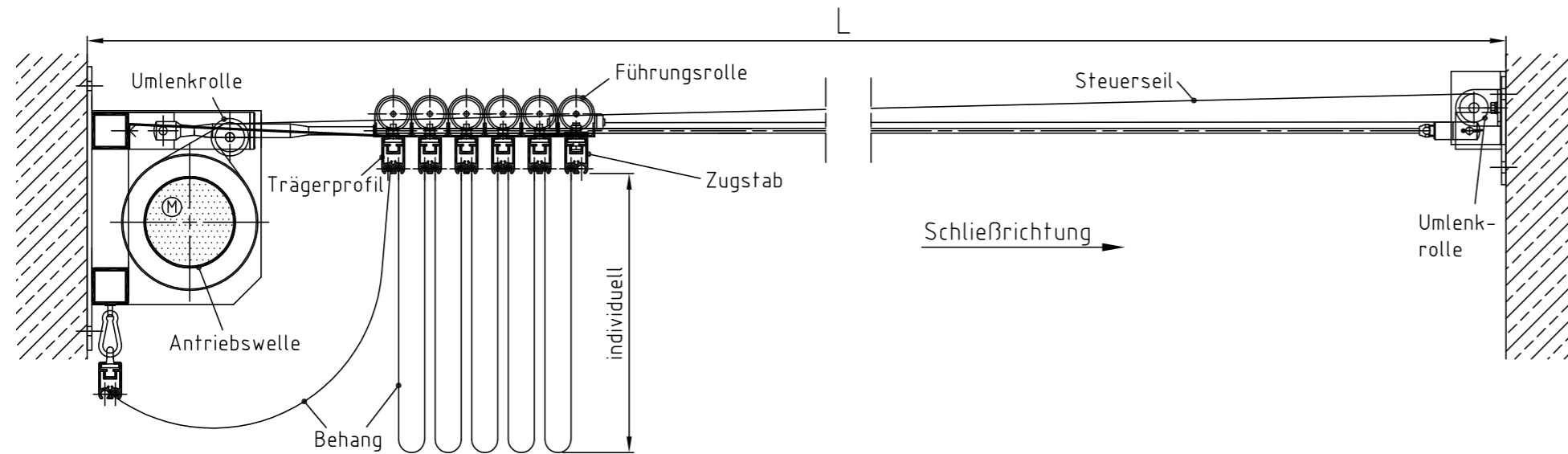
Zeichnung GZ-HR 200 – Querschnitt Systemskizze | ohne Maßstab | sämtliche Angaben in mm
