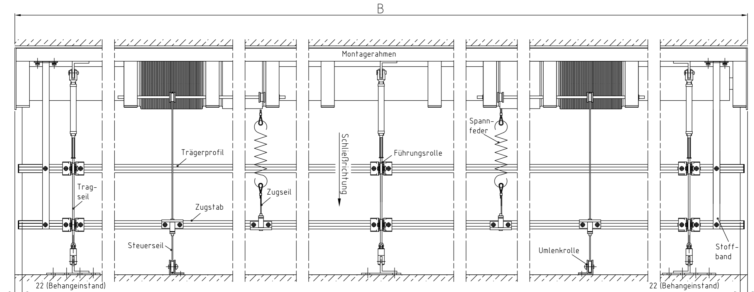
Zeichnung GZ-HR 200 – Draufsicht Systemskizze | ohne Maßstab | sämtliche Angaben in mm
