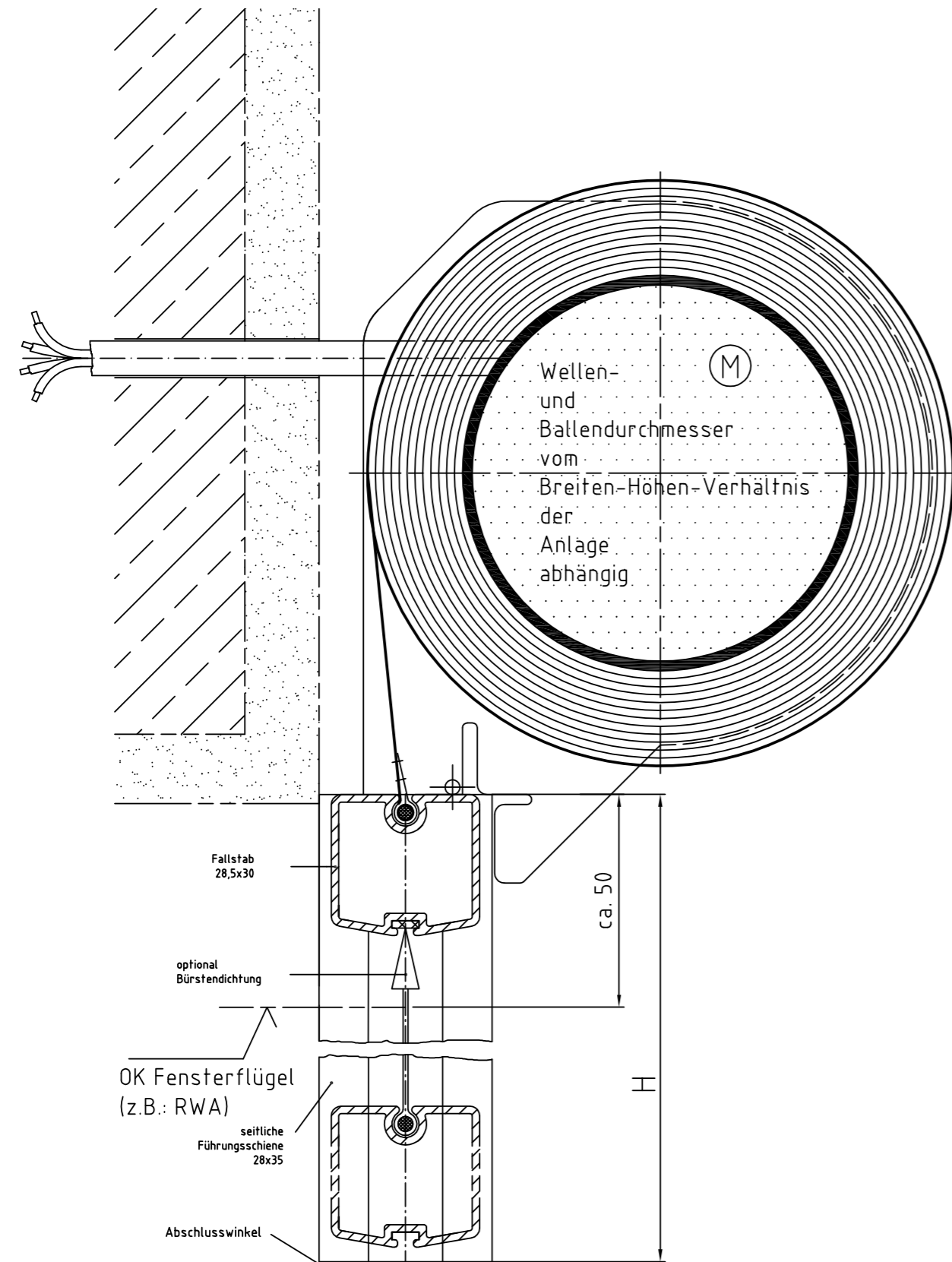
Zeichnung SM-ZIP-MO – Querschnitt Systemskizze | ohne Maßstab | sämtliche Angaben in mm
