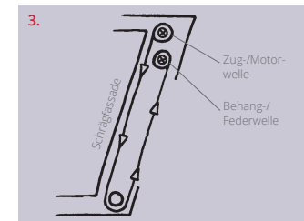
3. Vertikale Gegenzuganlage
