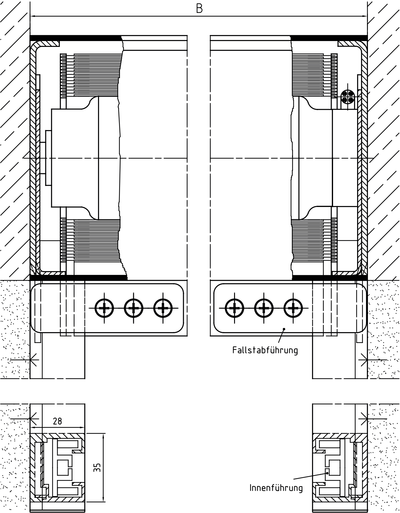
Zeichnung BS-ZIP-MQ3 – Querschnitt Systemskizze | ohne Maßstab | sämtliche Angaben in mm
