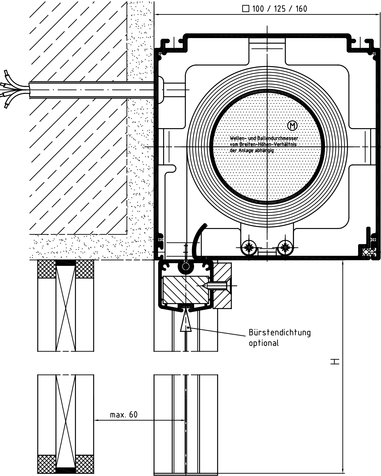
Zeichnung BS-ZIP-MQ3 – Längsschnitt Systemskizze | ohne Maßstab | sämtliche Angaben in mm
