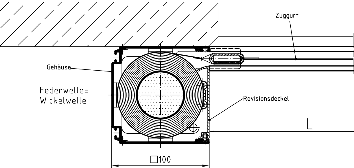
Zeichnung GZ-MQ 100 – Querschnitt Systemskizze | ohne Maßstab | sämtliche Angaben in mm
