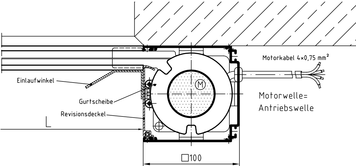
Zeichnung GZ-MQ 100 – Längsschnitt Systemskizze | ohne Maßstab | sämtliche Angaben in mm
