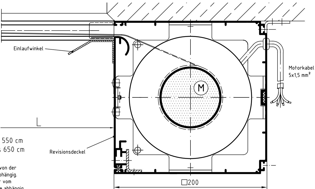
Zeichnung GZ-MQ 200 – Längsschnitt Systemskizze | ohne Maßstab | sämtliche Angaben in mm
