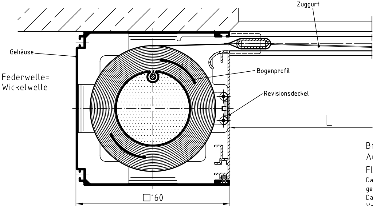
Zeichnung GZ-MQ 160 – Querschnitt Systemskizze | ohne Maßstab | sämtliche Angaben in mm
