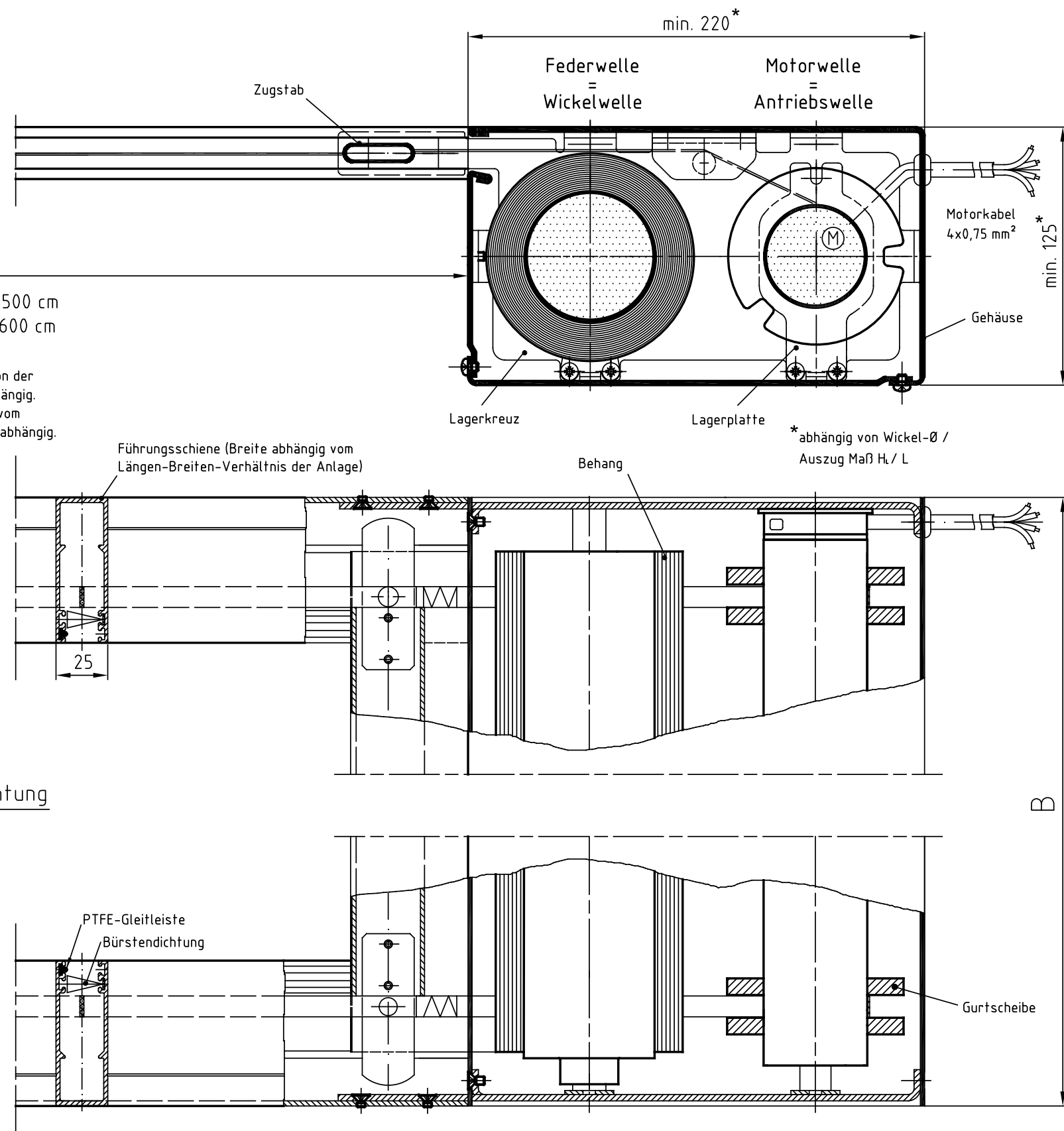
Zeichnung GZ-MQ 350 – Längsschnitt Systemskizze | ohne Maßstab | sämtliche Angaben in mm
