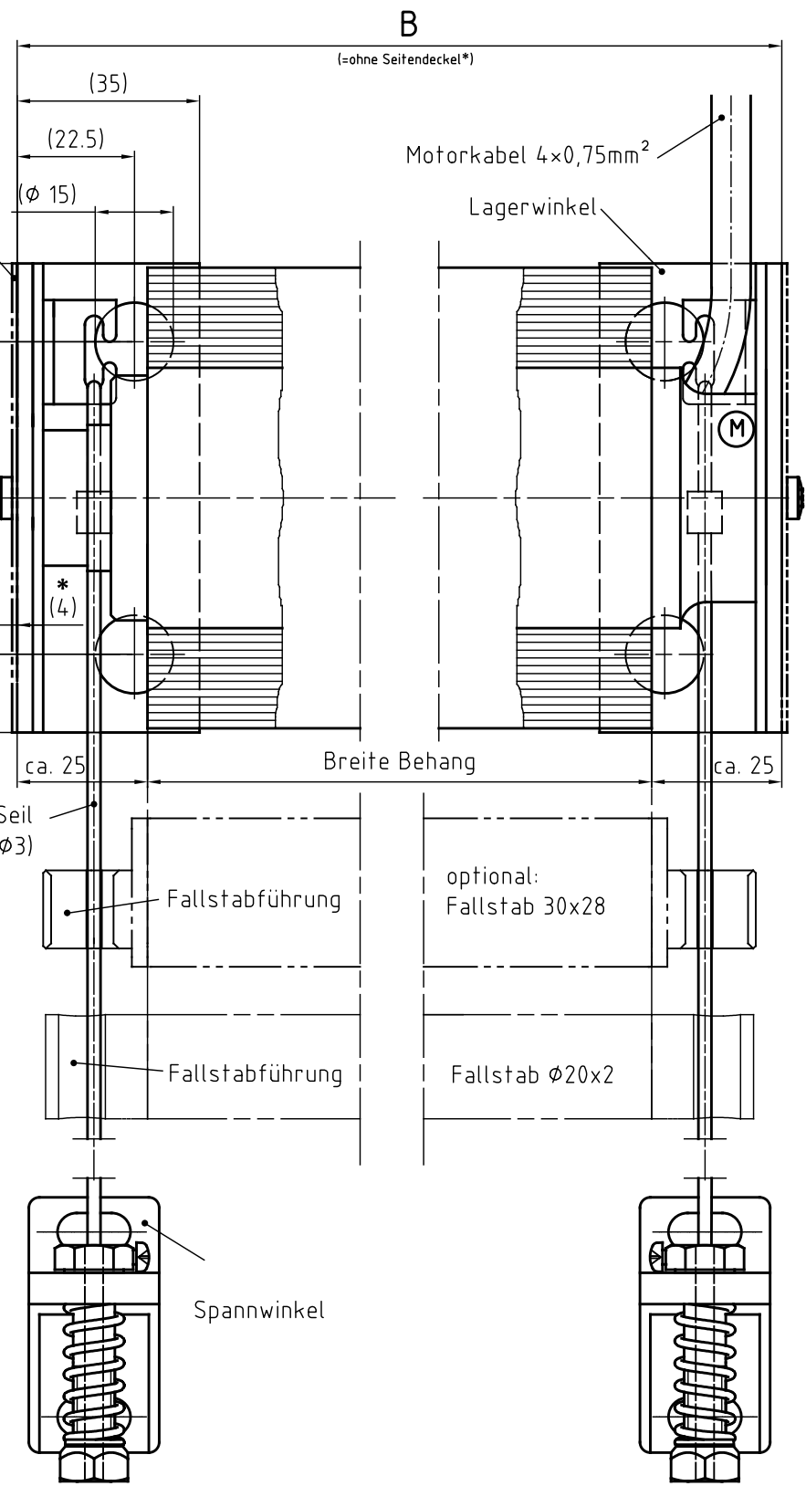
Zeichnung MO 100 – Längsschnitt Systemskizze | ohne Maßstab | sämtliche Angaben in mm
