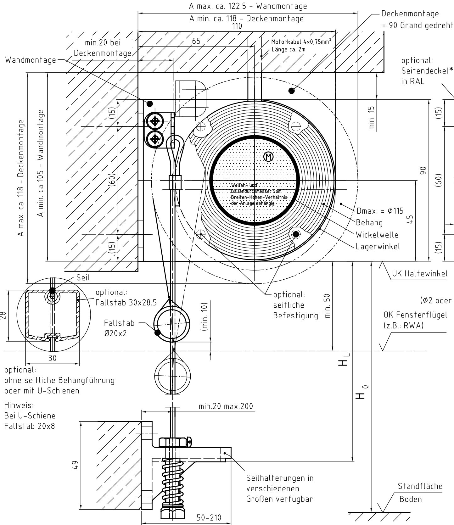
Zeichnung MO 100 – Querschnitt Systemskizze | ohne Maßstab | sämtliche Angaben in mm
