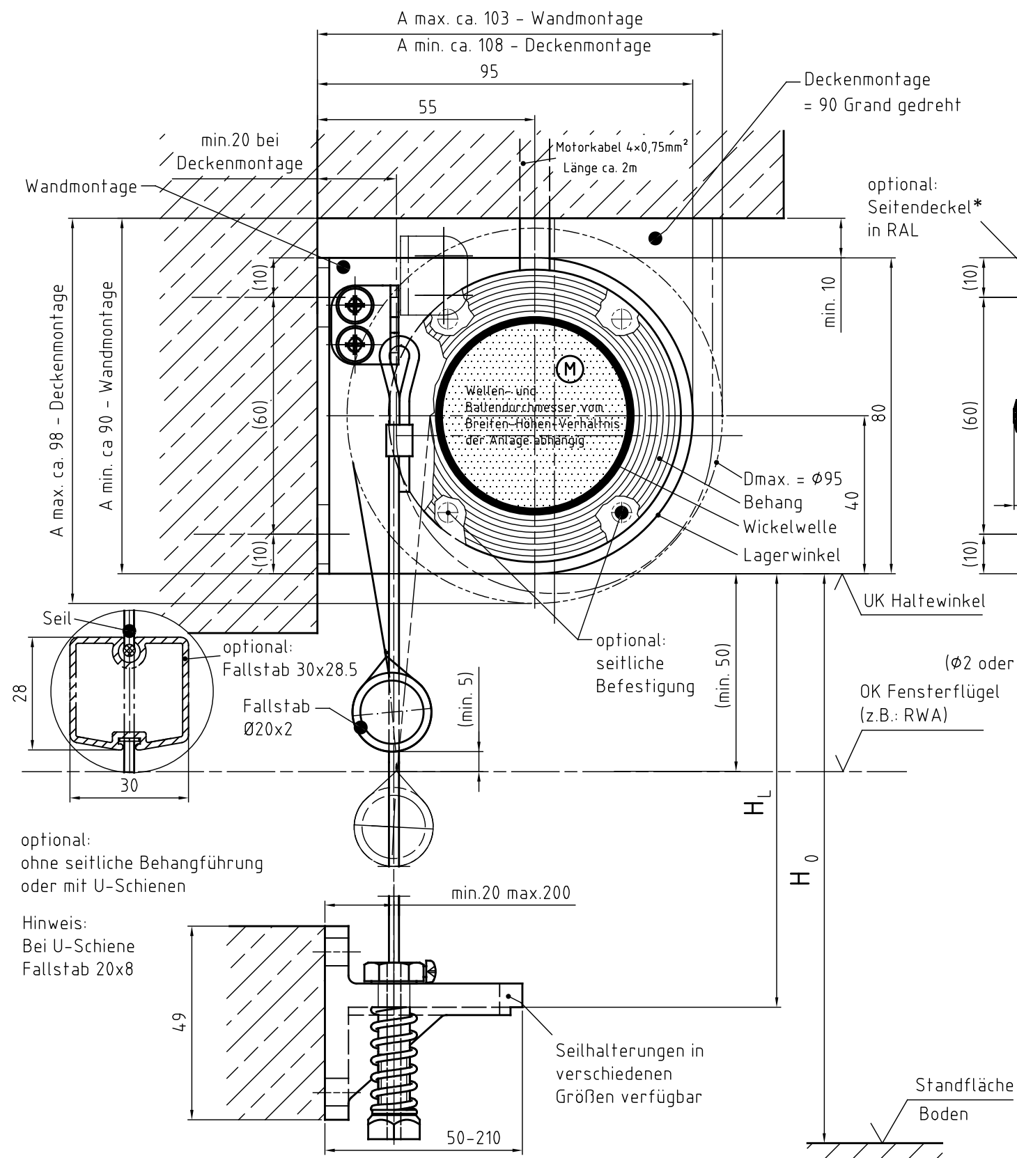
Zeichnung MO 80 – Querschnitt Systemskizze | ohne Maßstab | sämtliche Angaben in mm
